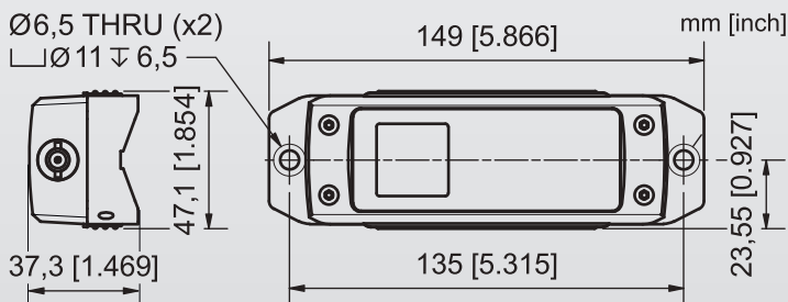
硬化鋼製精密プリズムベース ブラケット取付穴2個付き
