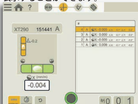
XT290のディスプレイ ライブ値およびグラフィックス
